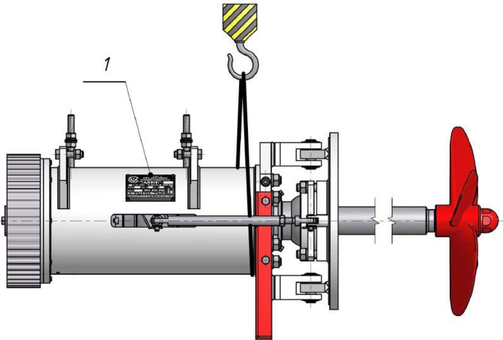
Схема строповки устройства "ТАЙФУН" без электродвигателя и плиты опорной
