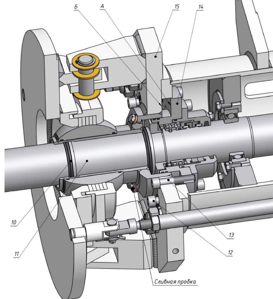
3 Фиксация вала гребного винта
