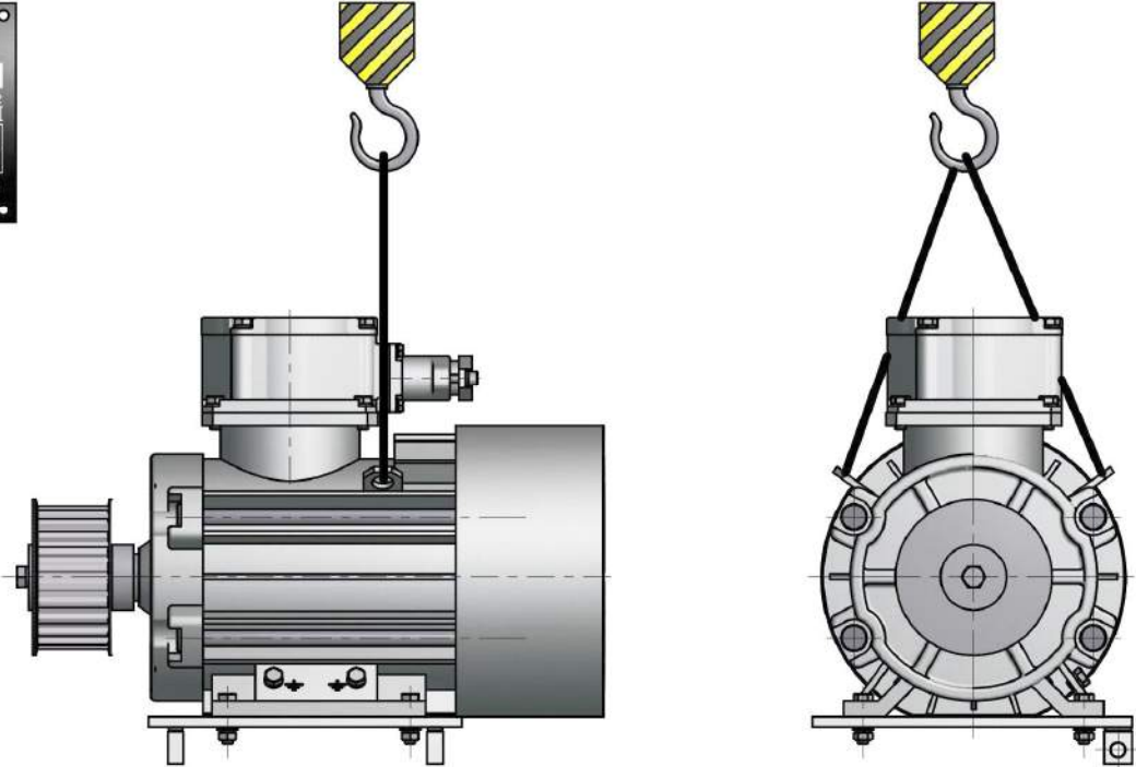
Схема строповки электродвигателя с плитой опорной
