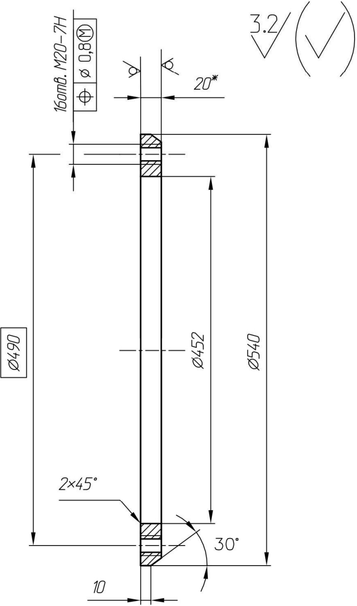
Монтажный фланец
