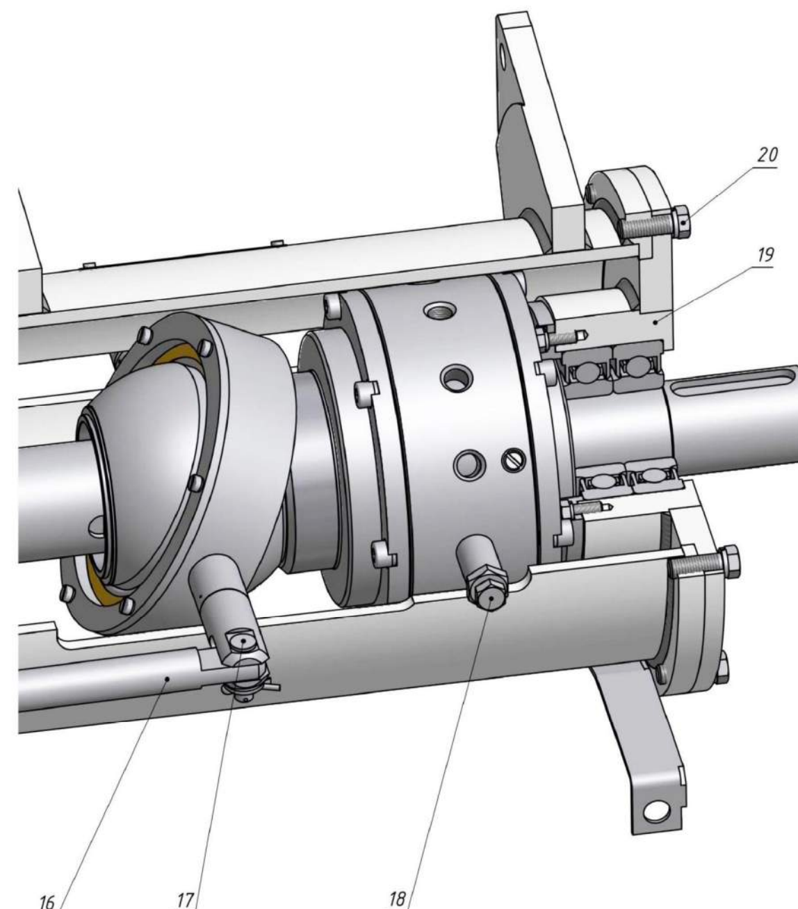
4 Демонтаж подшипниковой опоры и привода поворота
