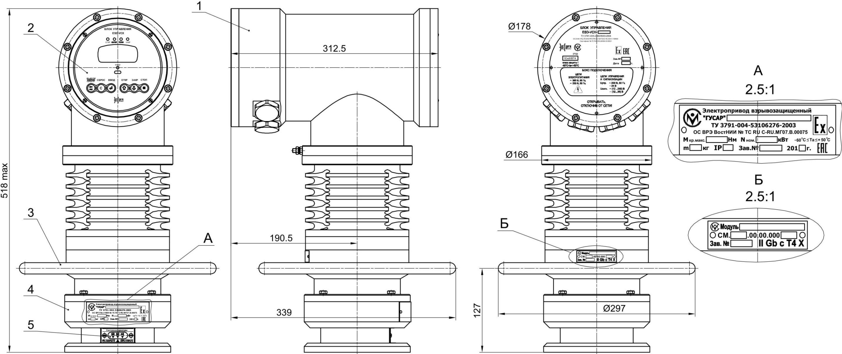
1. Блок управления ESD-VCX; 2. Встроенный пост управления; 3. Привод механизма ручного дублера; 4. Редуктор; 5. Указатель положения выходного звена;
