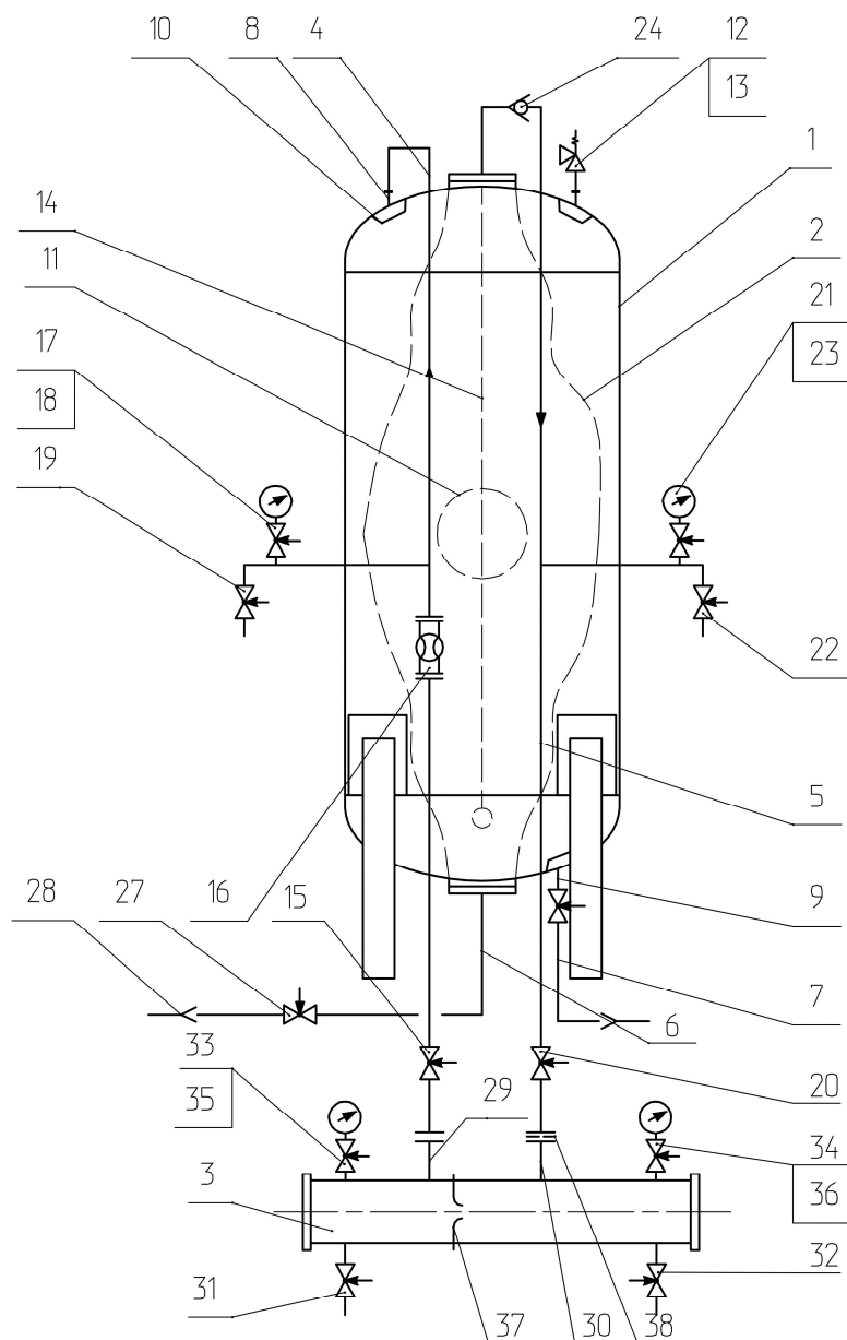
Рис. 1 . Схема принципиальная баков-дозаторов БДП "Гобсек"
