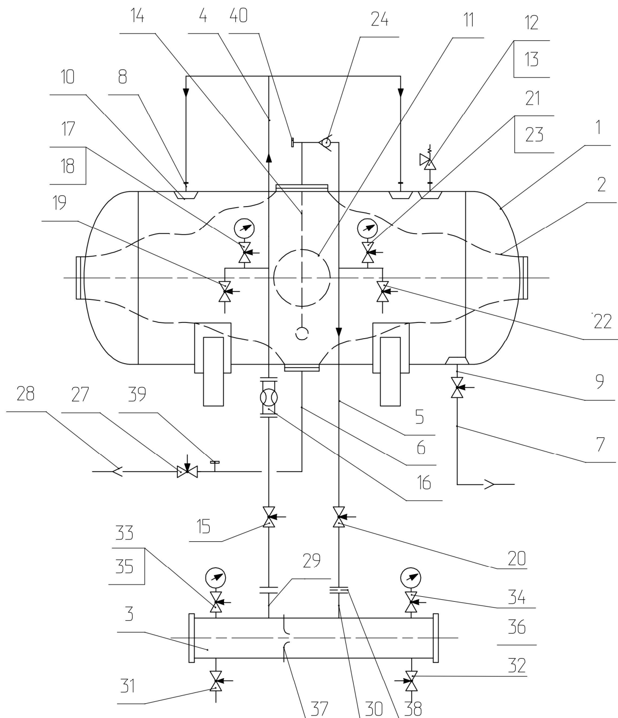
Рис. 1. Схема принципиальная баков-дозаторов БДП "Гобсек"
